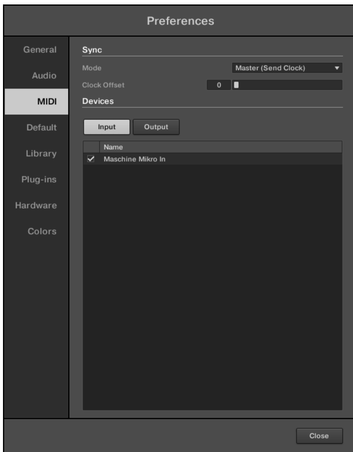
Preferencias – MIDI.
