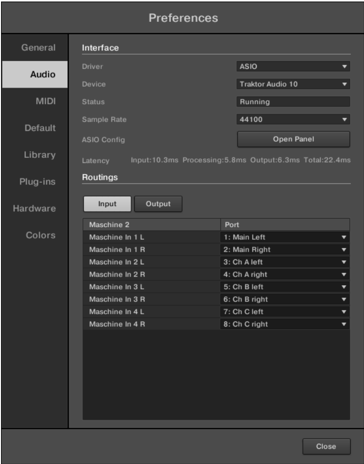
Preferencias – Audio
