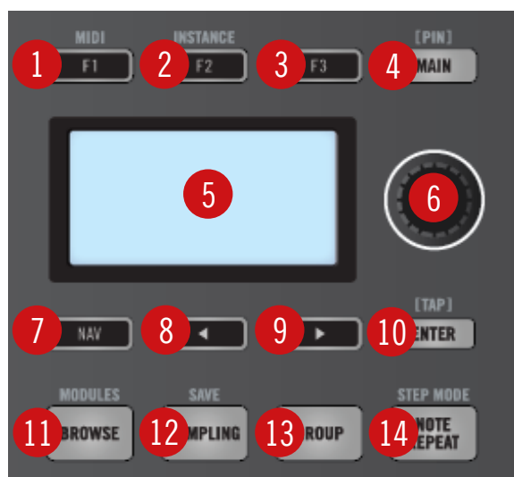
Vue d'ensemble de la section CONTROL.
